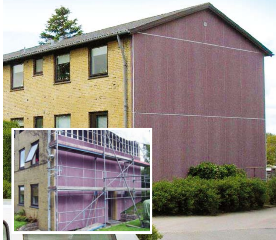
Gavl isolering af boligblok i Hjallesø.
